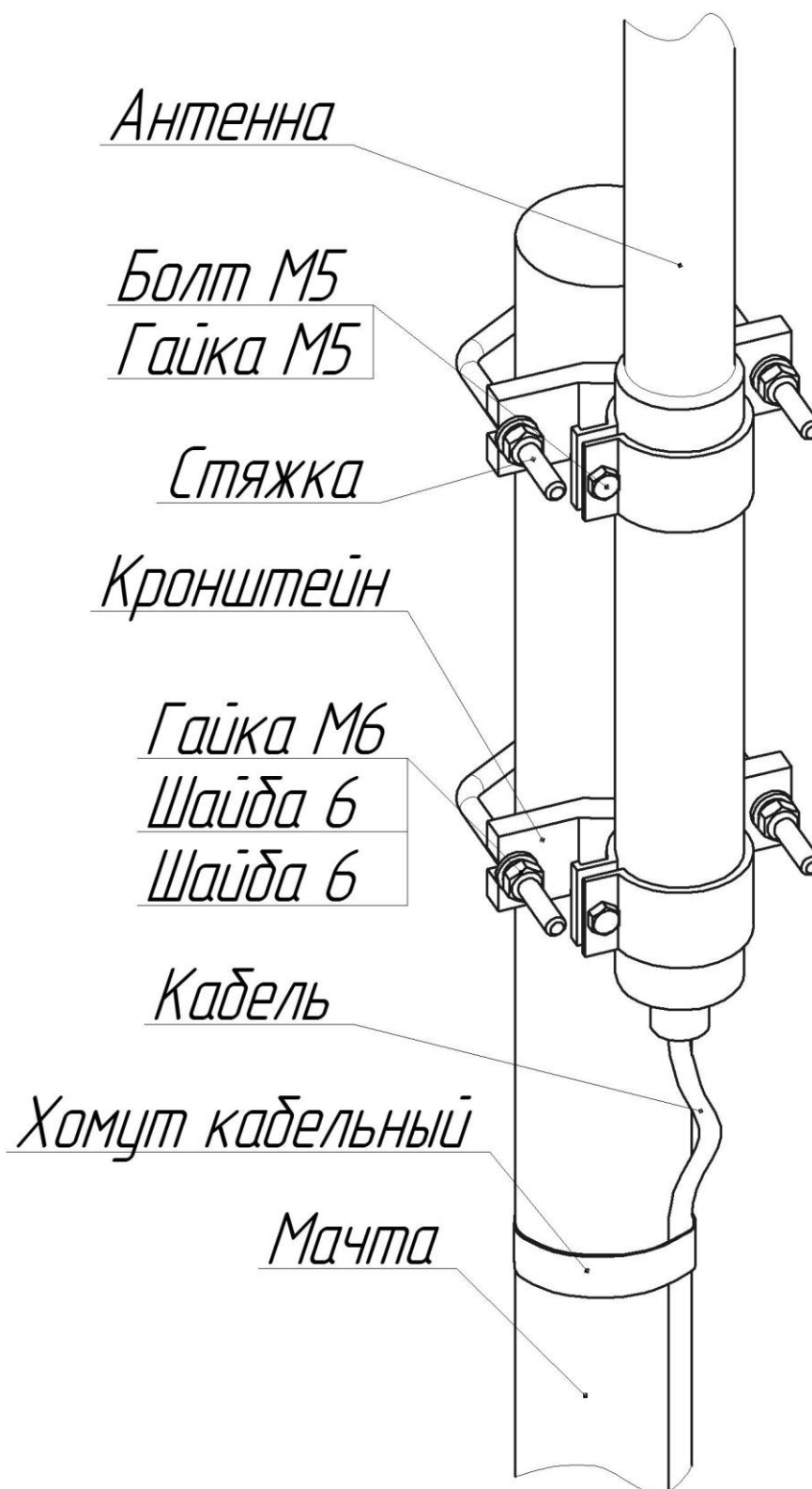
Рисунок 1 – Установка Комплекта Антенны АКБ-433 на мачте
