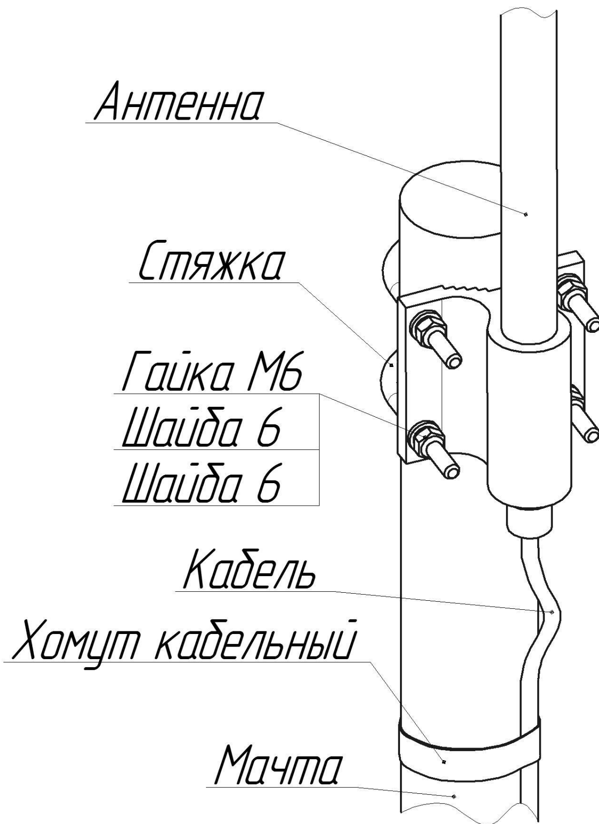
Рисунок 1 – Установка Комплекта Антенны АКМ-433 на мачте
