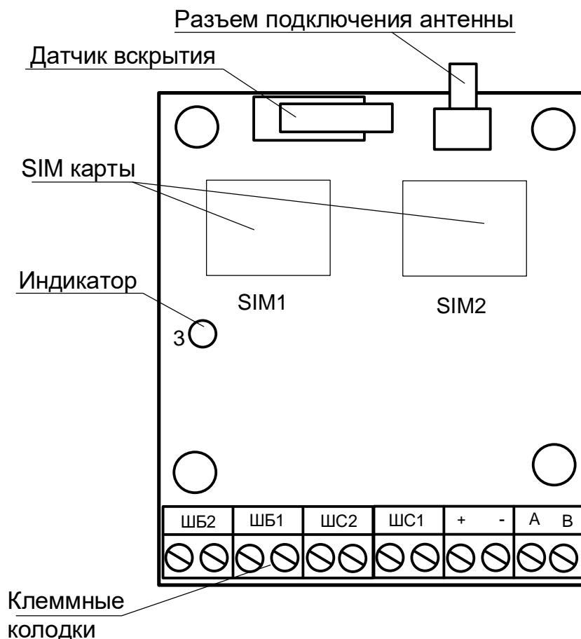
Рисунок 1 – Панель GSM-ПРМ
