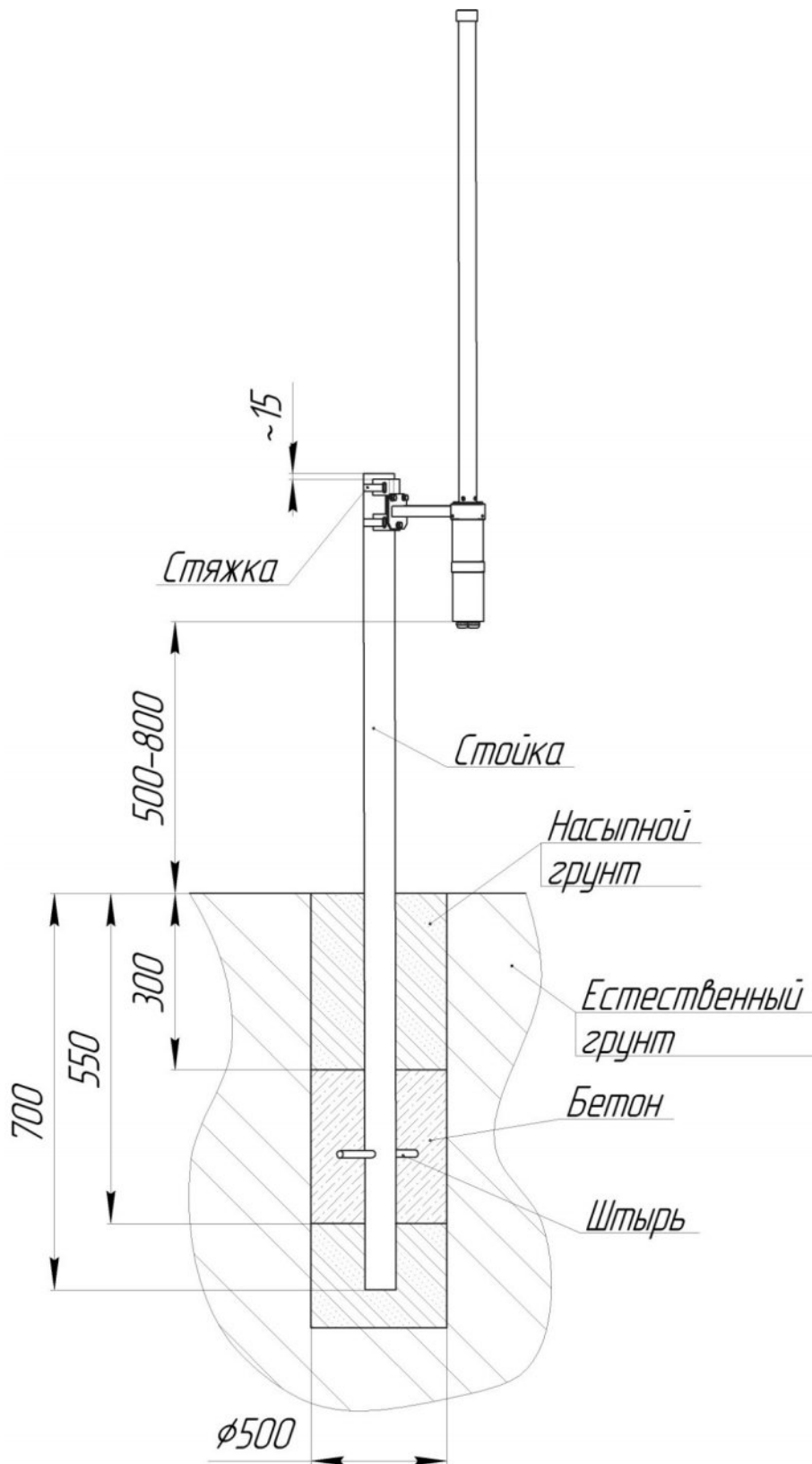
Рисунок 2 – Установка блоков извещателя
