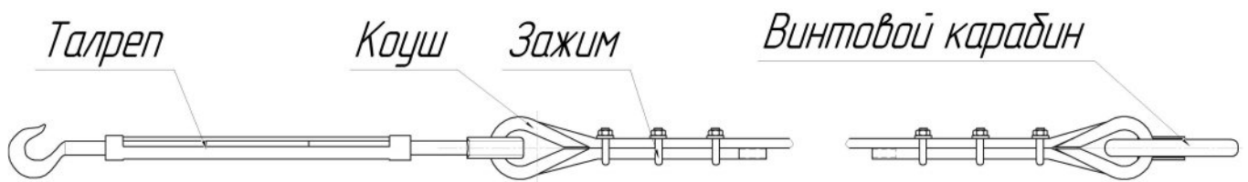
Рисунок 6 – Оттяжка
