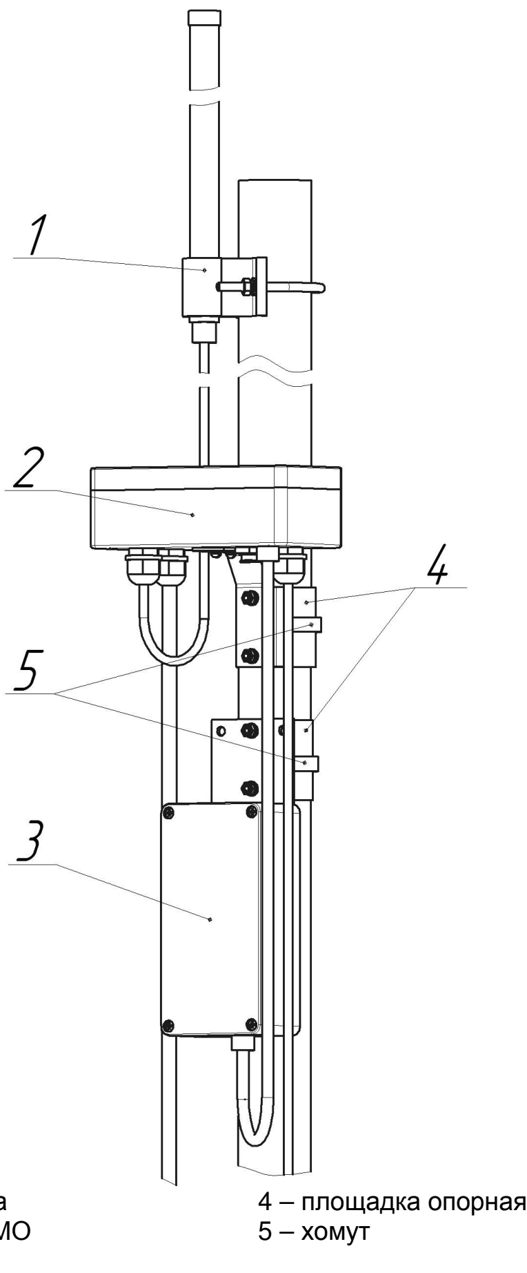
Рисунок 2 – Крепление на опоре
